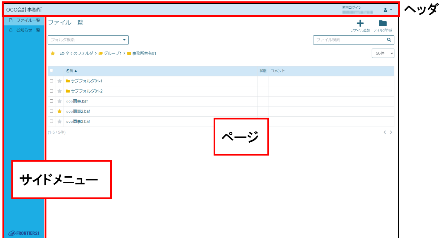
図 2.4: 画面構成
