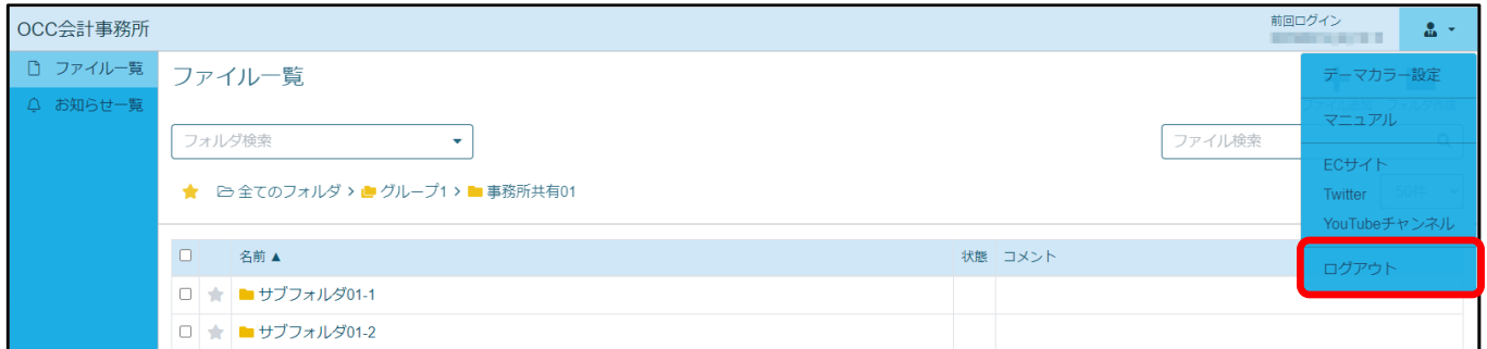
図 2.3: [ログアウト]
